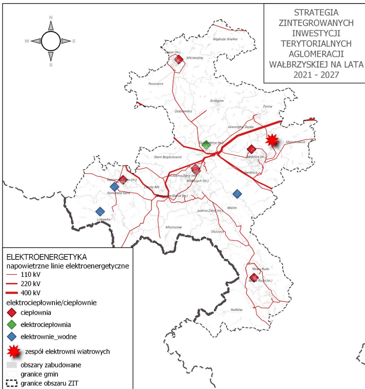
Mapa 54. Sieci i infrastruktura elektroenergetyczna
